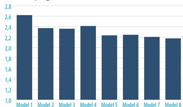
Figuur 5. Odds-ratio per geschat model.
